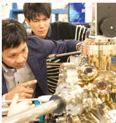
光電子分光法による電子状態測定
