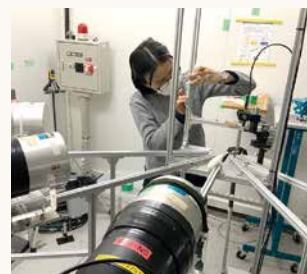
光中性子測定のための検出器設置の様子
