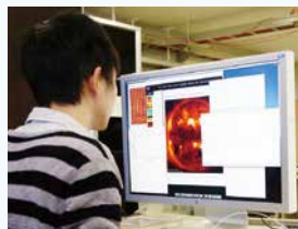
人工衛星観測で得られたデータの解析
