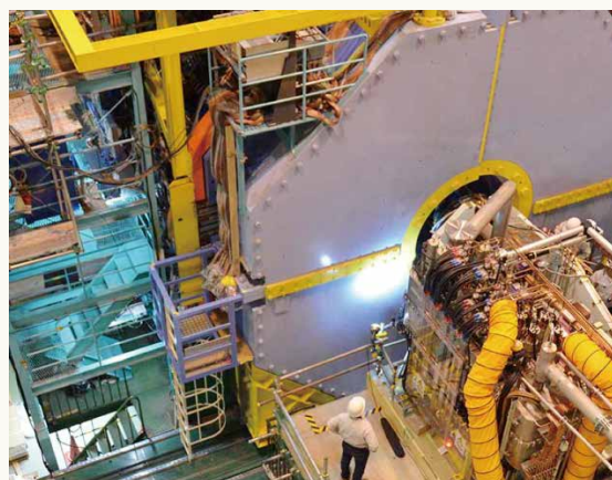
新物理の発見を目指して運転を開始した Belle II 測定器 ©KEK
