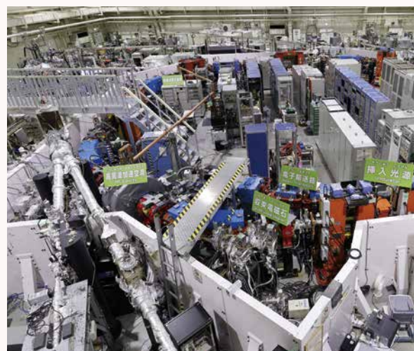
極端紫外光シンクロトロン放射光研究施設 UVSOR-III
